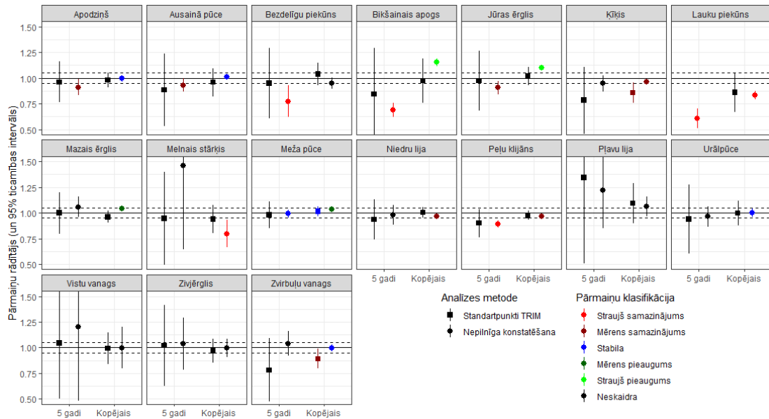
3.4.1. attēls. Plēsīgo putnu populāciju pārmaiņu rādītāju, kas iegūti ar dažādām metodēm, klasifikācija. Melnā horizontālā līnija nozīmē stabilu populāciju, raustītās līnijas robežlielumus klasifikācijas statistiskajam nozīmīgumam.
