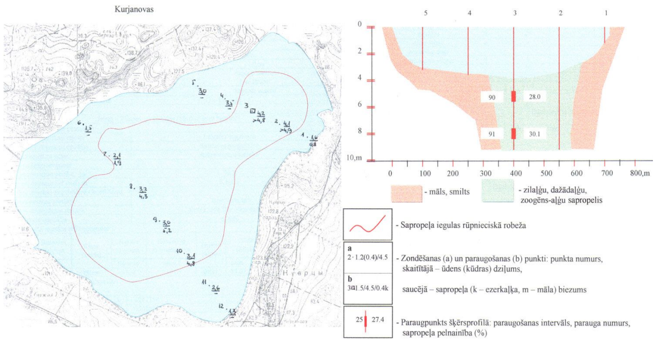
6.attēls. Kurjanovas ezera nogulumu shēma (VĢD, 1999).
