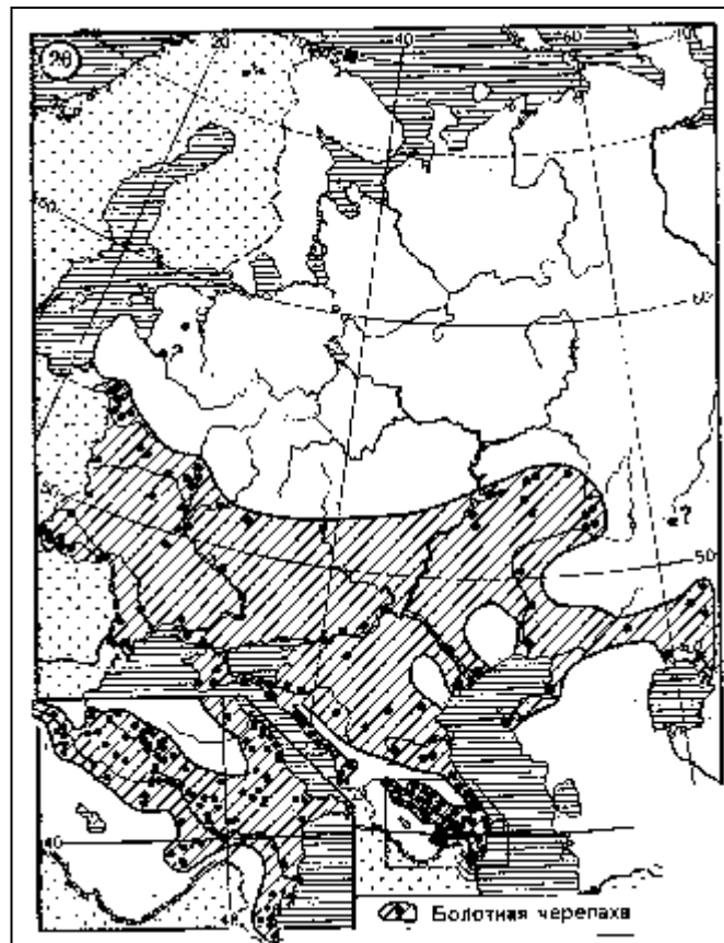
33.att. Eiropas purva bruņurupuča areāls bijušajā Padomju Savienībā (Bannikov et al. 1977)
